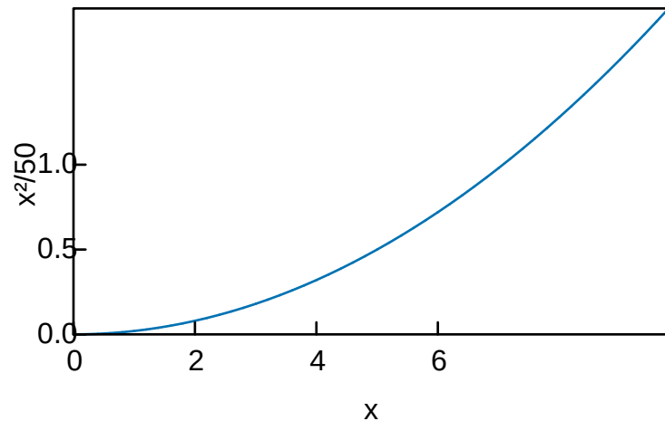
Quadratic Function
