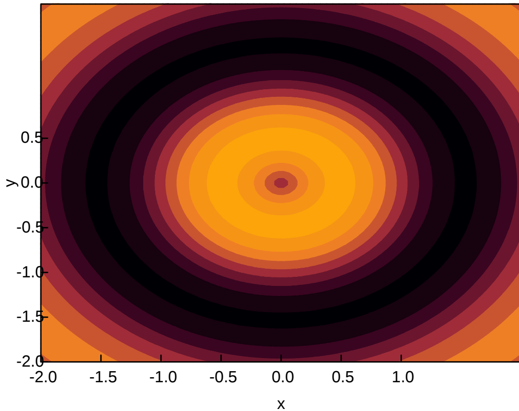
Ripple Function - Inferno Colormap
